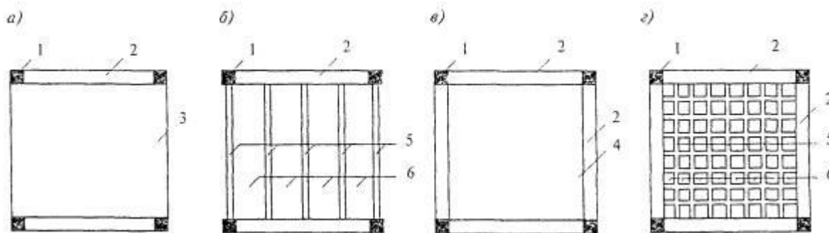
а, б - балки и стены в одном направлении, в, г - балки и стены в двух направлениях;
