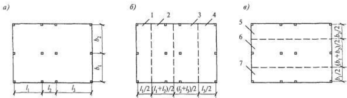
a - общая схема; б - поперечная схема; в - продольная схема;
