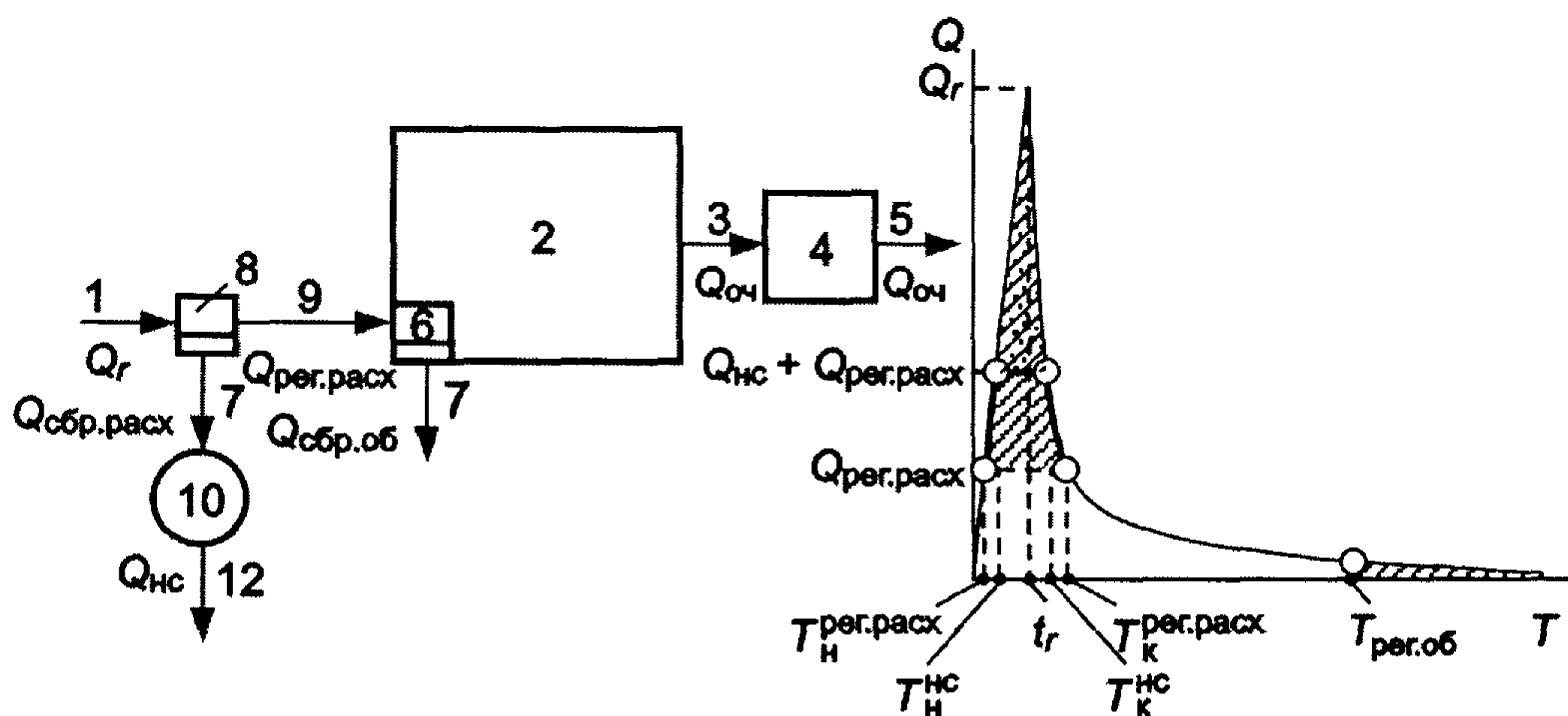
Рис. 5. Схема перекачки избыточной части зарегулированного по расходу дождевого стока □ часть объема дождя, поступающего в аккумулирующий резервуар для последующей очистки; ▨ рабочий объем резервуара насосной станции; ▩ часть объема дождя, отводимого в водный объект без очистки
