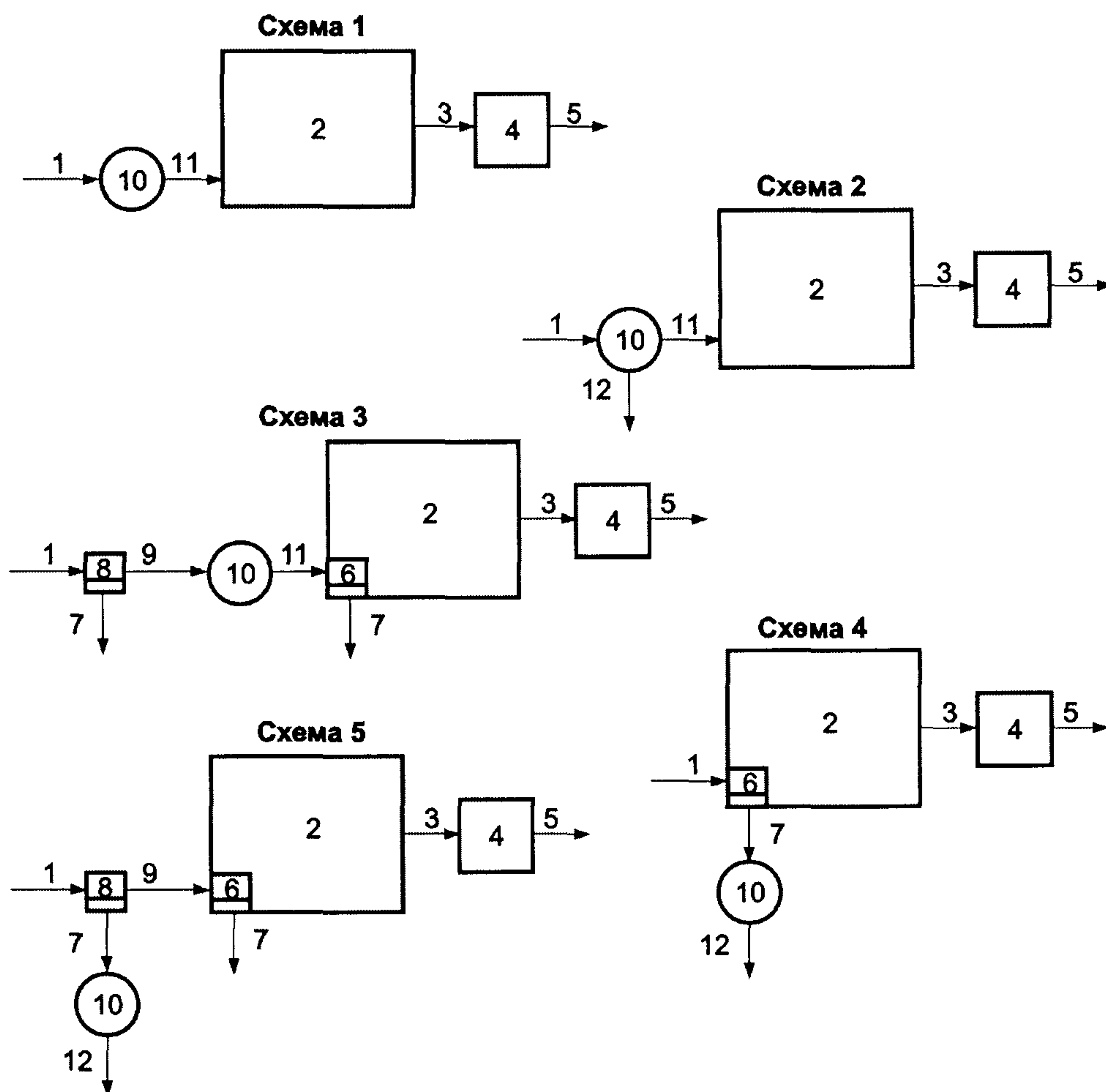
Рис. 2. Основные схемы перекачки дождевого стока
