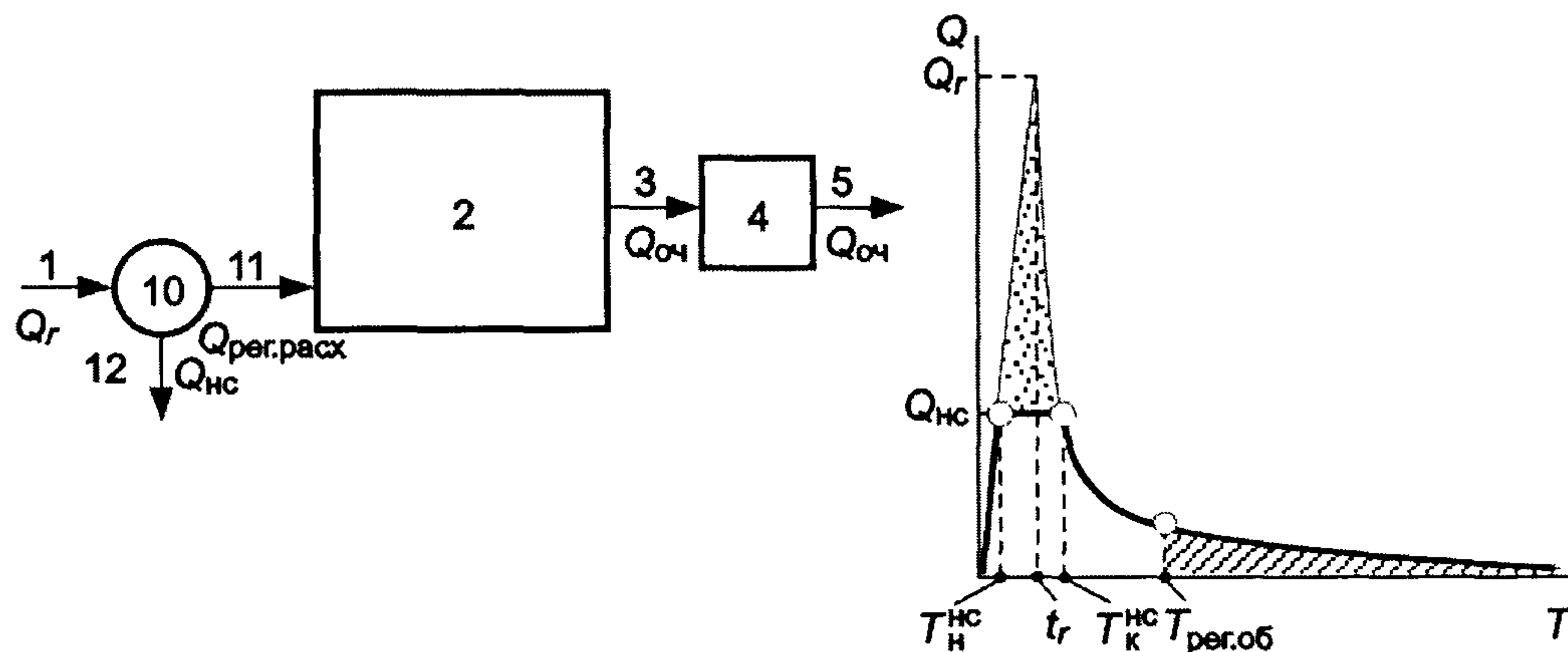
Рис. 2. Схема перекачки избыточной части зарегулированного по объему дождевого стока 1 – 5, 10, 11 – см. рис. 1; 12 – напорный трубопровод перекачки избыточного стока; □ часть объема дождя, поступающего в аккумулирующий резервуар для последующей очистки; ▨ часть объема дождя, отводимого в водный объект без очистки; ▩ рабочий объем резервуара насосной станции
