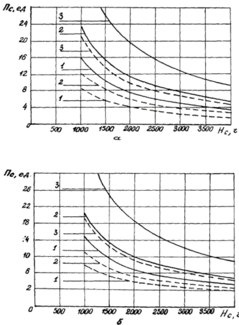
Рис. 4. Пропускная способность одного ангарного места стоянки для перспективных воздушных судов Ил-96 (1), Ту-204 (2) и Ми-26 (3):
