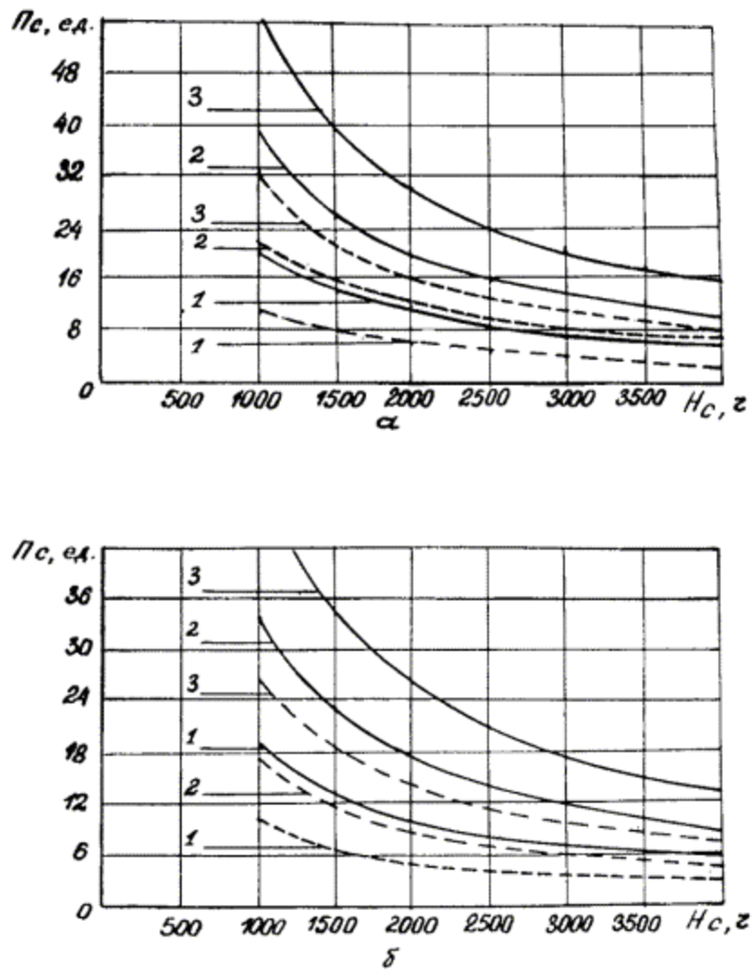
Рис. 5. Пропускная способность одного ангарного места стоянки самолетов, находящихся в эксплуатации, Ил-86 (1), Ту-154 (2) и Як-42 (3):
