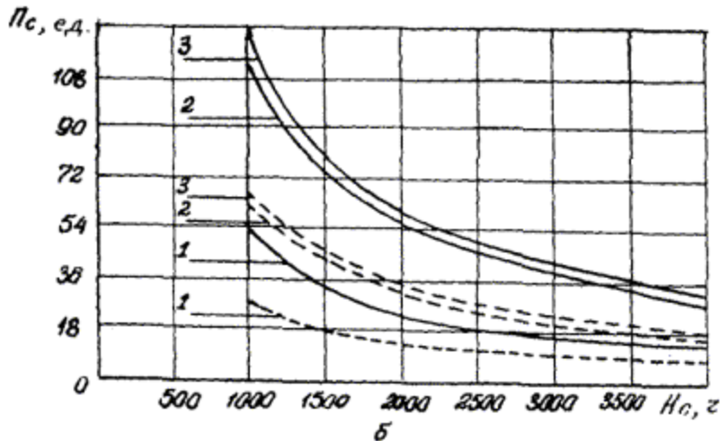
Рис. 6. Пропускная способность одного ангарного места стоянки воздушных судов, находящихся в эксплуатации, Ми-8 (1), Як-40 (2) и Л-410 (3):
