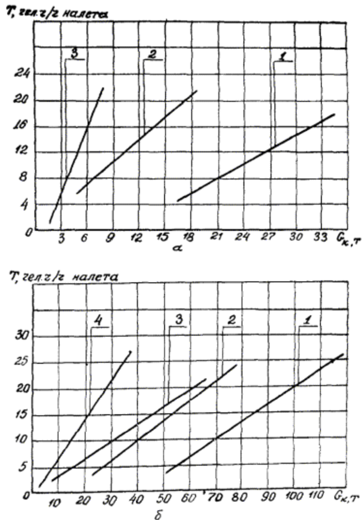
Рис. 3. Удельная трудоемкость технического обслуживания ВС в зависимости от массы конструкции вертолетов I - III классов (а) и самолетов I - IV групп (б):
