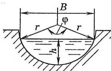
Рисунок Л.4 – Схема канала кругового сечения
