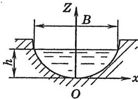
Рисунок Л.3 – Схема канала параболического сечения
