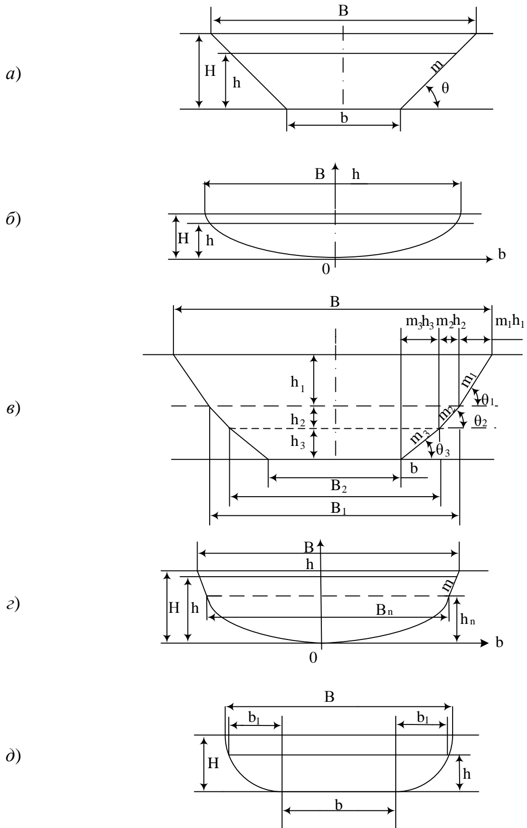
a – трапецидальная; б – параболическая; в – полигональная; г – комбинированная; д – параболическая с донной вставкой
