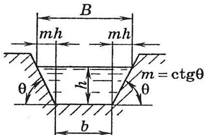
Рисунок Л.1 – Схема канала трапецеидального сечения
