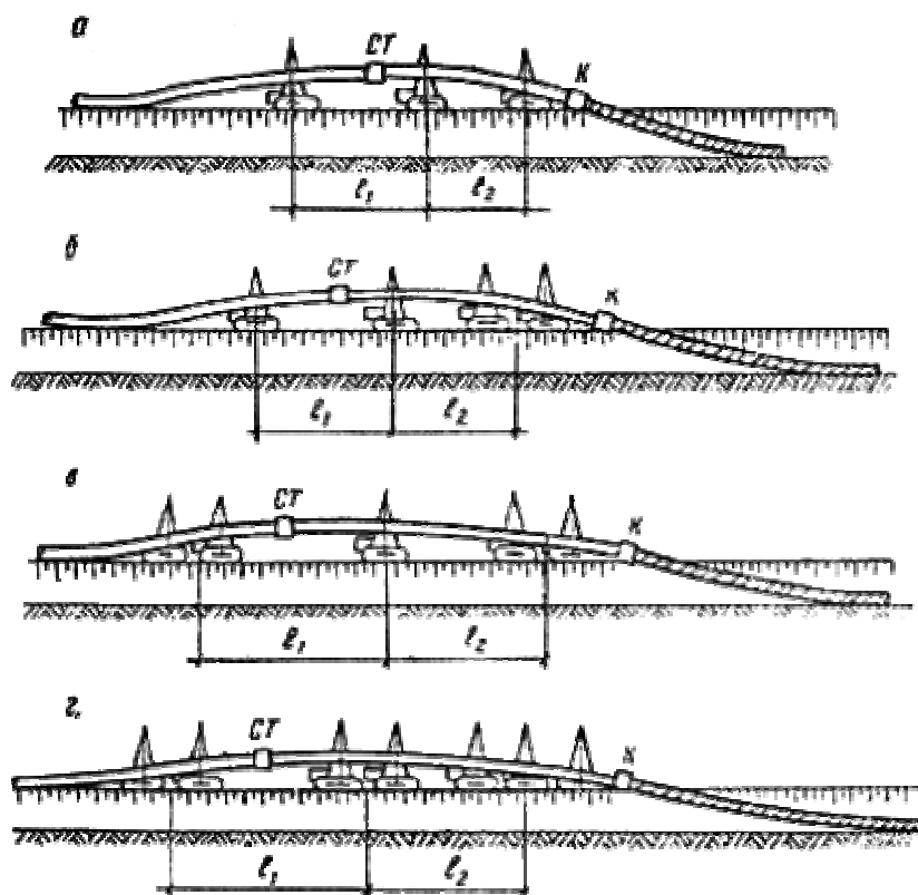
Рис. 10. Схемы расстановки трубоукладчиков и машин в изоляционно-укладочной колонне при совмещенном способе производства работ для трубопроводов различных диаметров:
