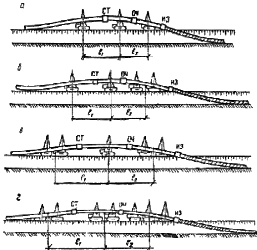
Рис. 9. Схемы расположения трубоукладчиков и машин в изоляционно-укладочной колонне при совмещенном способе производства работ для трубопроводов различных диаметров:
