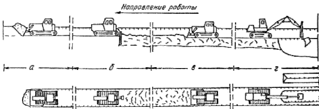
Рис. 6. Схема разработки траншеи в мерзлом грунте с предварительным рыхлением его механическим рыхлителем:
