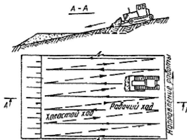
Рис. 2. Схема разработки полок на склонах поперечными проходами бульдозера
