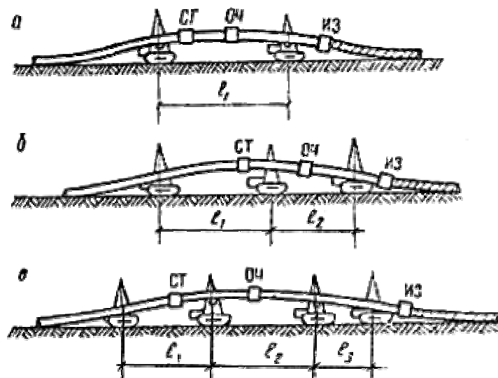
Рис. 12. Схемы расположения трубоукладчиков и машин в изоляционно-укладочной колонне для трубопроводов различных диаметров:
