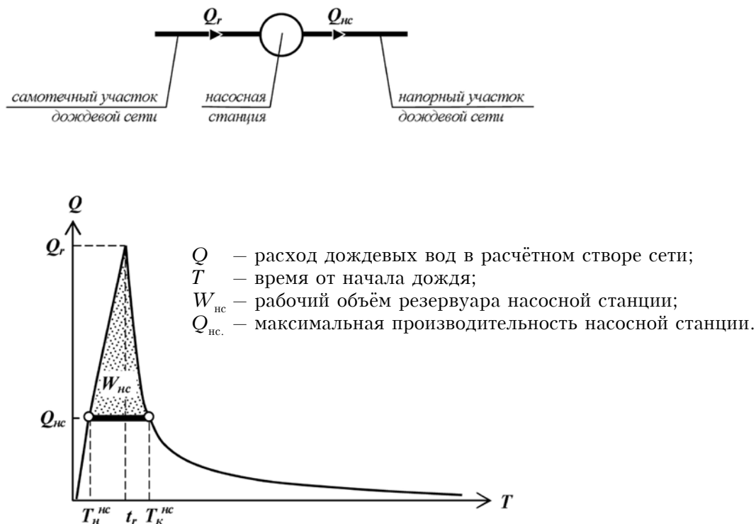
Рисунок 1. Схема и расчётный гидрограф перекачки незарегулированного стока
