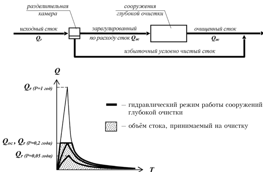
Рисунок 4. Схема и гидрограф гидравлического режима работы очистных сооружений проточного типа
