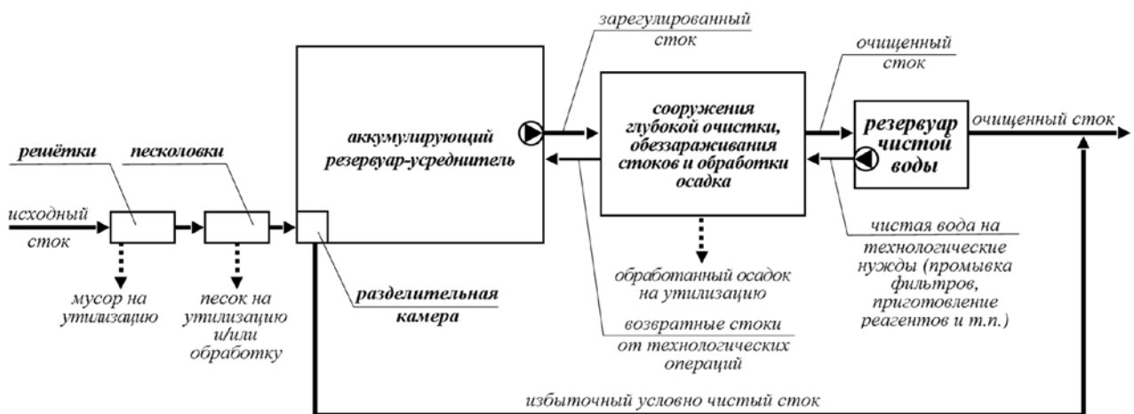
Схема 3 – с осаждением тяжёлых механических примесей (песка) перед разделением и аккумуляцией стока
