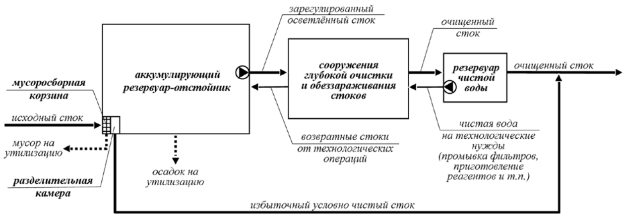
Схема 1 – с предварительным осветлением стока в аккумуляционном резервуаре
