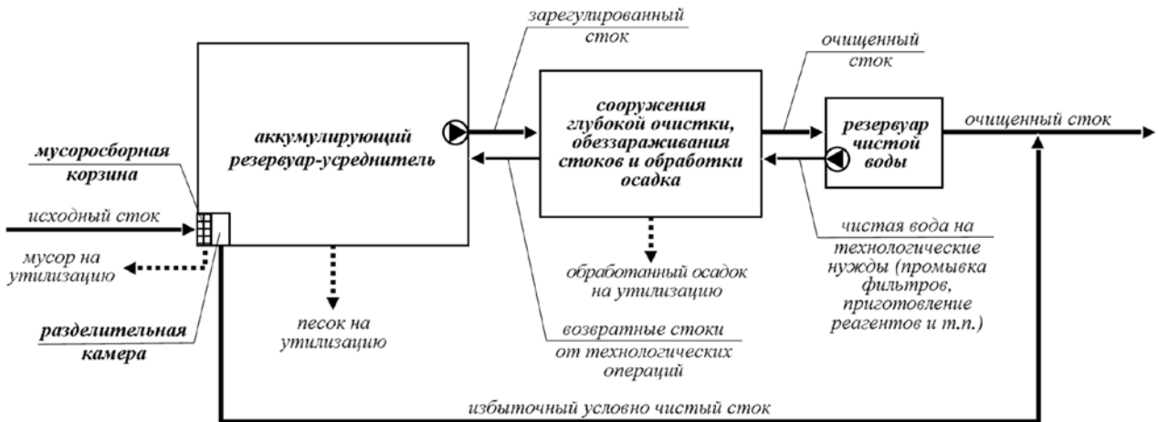
Схема 2 – с осаждением тяжёлых механических примесей (песка) в аккумуляционном резервуаре
