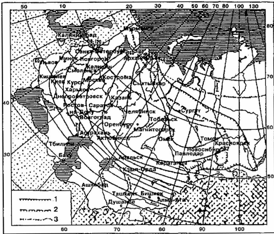
Рис. 4.4. Карта изолиний глубины промерзания Z_{пр(ср)} грунтов на территории СНГ:
