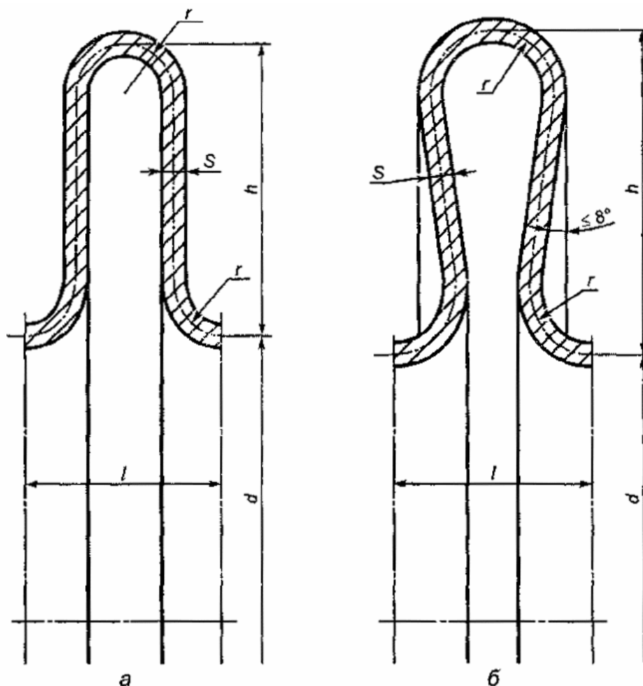
Рисунок 1 - Модели компенсаторов
